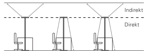
Direkt- und Indirektlicht sind getrennt schalt- und dimmbar.
